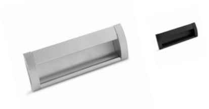
Материал: алюминий/пластик Размеры: 42x35x140,5 мм
