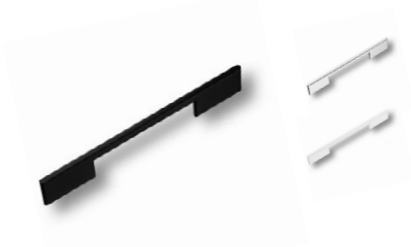
Материал: алюминий Размеры: 30x7x220 мм
